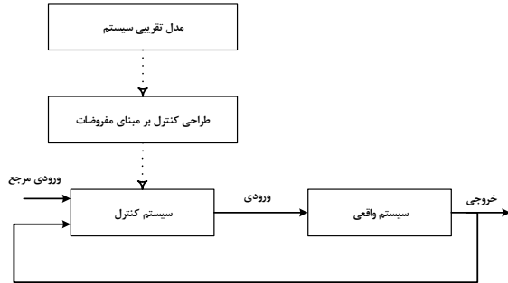
شکل ۱: ساختار طراحی سیستم‌های کنترل مدل پایه
