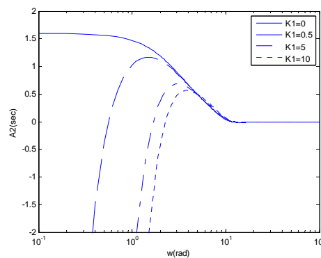
شکل ۱۰: شرط پایداری A_2 به ازای K_2 = 4, \alpha = 0, \tau_1 = 0.3 و مقادیر مختلف K_1 و \zeta = 0.5, \omega_n = 10
