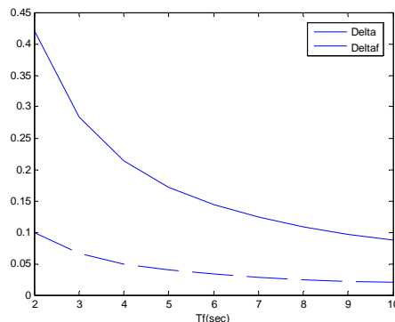
شکل ۹: نمایش \delta و \delta_f بر حسب زمان پرواز به ازای K_1 = 2, \omega_n = 10 و \zeta = 0.5, \tau_1 = 0.3, K_2 = 4
