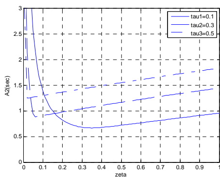
شکل ۸: شرط پایداری A_2 بر حسب \zeta به ازای K_1 = 0.5, \alpha = 0 و مقادیر مختلف \tau_1 و K_2 = 4, \omega_n = 10
