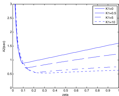
شکل ۷: شرط پایداری A_2 بر حسب \zeta به ازای K_2 = 4, \alpha = 0 و مقادیر مختلف K_1 و \tau_1 = 0.2, \omega_n = 10
