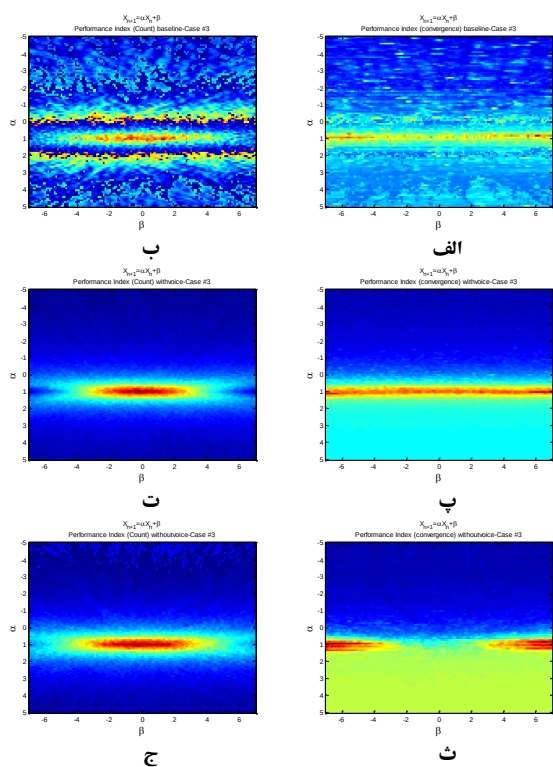
شکل ۹. بررسی صفحه پوانکاره بهینه یک بعدی در اتیسم (فضای بازسازی شده‌ی نسبی تگر) سمت چپ معیار بیشترین تعداد برخورد، سمت راست معیار بیشترین بسط سیگنال
