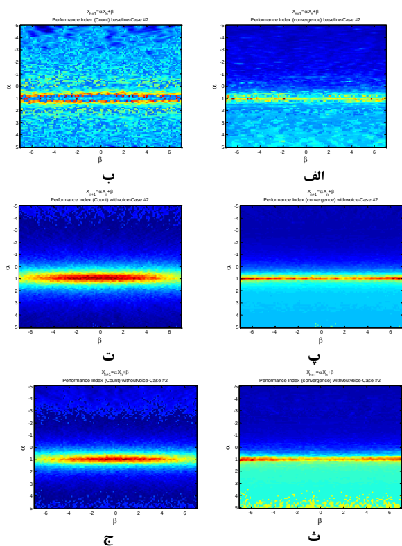
شکل ۸. بررسی صفحه پوانکاره بهینه یک بعدی در سالم (فضای بازسازی شده‌ی نسبی تگر) سمت چپ معیار بیشترین تعداد برخورد، سمت راست معیار بیشترین بسط سیگنال
