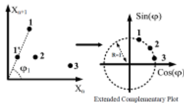
شکل ۵. طریقه اعمال نمودار مکمل توسعه یافته
