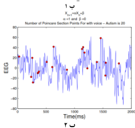
شکل ۲. قطع پوانکاره سیگنال EEG با خط Y=X در فضای بازسازی شده نسبی تگر و حوزه زمان الف. سالم ب. ASD
