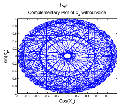
شکل ۴. بازنمایی سیگنال EEG کودک ASD به روش نمودار مکمل استاندارد برای سیگنال با طول ثابت (۸ ثانیه با فرکانس ۲۵۶) و شرایط مختلف روی دو کانال C3 (نمایشده نیمکره چپ که در شکل‌ها شماره ۱ دارند) و C4 (نمایشده نیمکره راست که در شکل‌ها شماره ۲ دارند) الف. وضعیت زمینه ب. وضعیت با صدا پ. وضعیت بدون صدا
