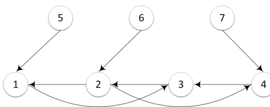
شکل ۱: گراف ارتباطات
