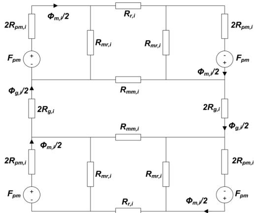
شکل ۳. مدار معادل مغناطیسی ژنراتور برای نصف زوج قطب
