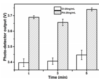
شکل ۱۰: خروجی ولتاژ دیتکتور نوری در حضور مواد مورد نظر
