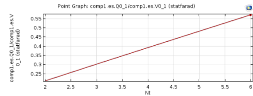
شکل ۳۸: نمودار مربوط به تغییرات میزان خازن شانه ای بر حسب تغییرات تعداد شانه ها
