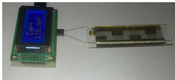
شکل ۶۷: مدار و ساختار ریزسیالی ساخته شده در هنگام انجام آزمایش
