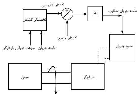
شکل ۳: بلوک دیاگرام طرح کنترلی گشتاور بار فوکو
