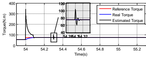
شکل ۱۰: نتایج شبیه‌سازی کنترل کننده در حالت دوم. الف- گشتاور ب- جریان تحریک ج- سرعت دورانی دینامومتر
