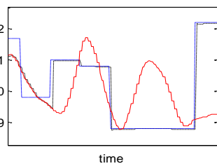
شکل ۹- تخمین زاویه سمت با فیلتر تکمیلی، سوئیچ از مغناطیس سنج به GPS در فاز حرکت سطحی
