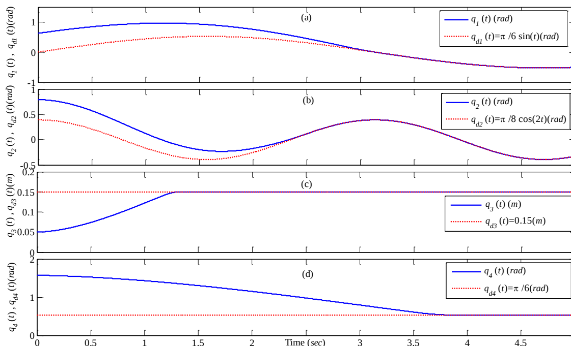
شکل ۶. پاسخ‌های زمانی متغیرهای پیکربندی مفاصل ربات SCARA با اعمال گشتاورهای پیشنهادی دسته دوم و فرض در نظر گرفتن غیرخطی‌سازهای شعاعی. (a): پاسخ‌های زمانی q_1(t) و q_2(t) ; (b): پاسخ‌های زمانی q_2(t) و q_{d2}(t) ; (c): پاسخ‌های زمانی q_3(t) و q_{d3}(t) ; (d): پاسخ‌های زمانی q_4(t) و q_{d4}(t)
