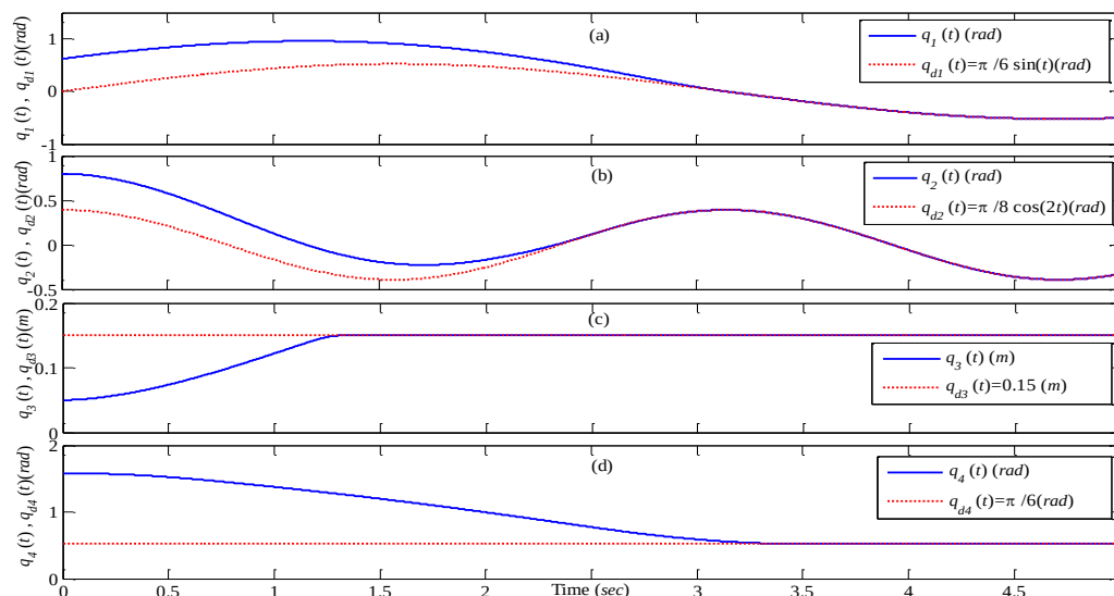
شکل ۱۰. پاسخ‌های زمانی پی‌گیری مفصل‌های ربات SCARA با اعمال گشتاورهای پیشنهادی دسته چهارم و فرض در نظر گرفتن غیرخطی‌سازهای ناحیه مرده. (a): پاسخ‌های زمانی
