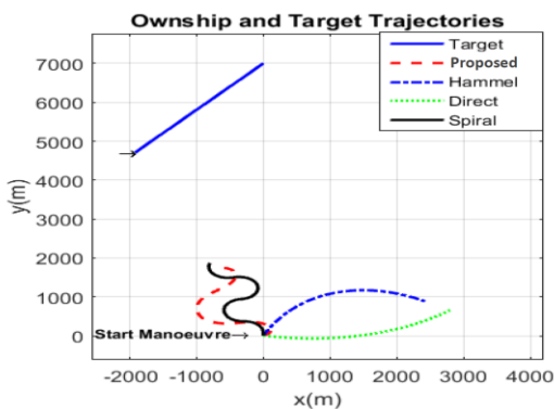
شکل ۷- ب: مسیر رویتگر هدف بدون مانور (فاصله ۷km)
