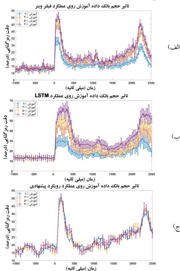
شکل ۱۱: تأثیر کاهش حجم داده آموزش برای (الف) فیلتر وینر، (ب) LSTM و (ج) روش پیشنهادی
