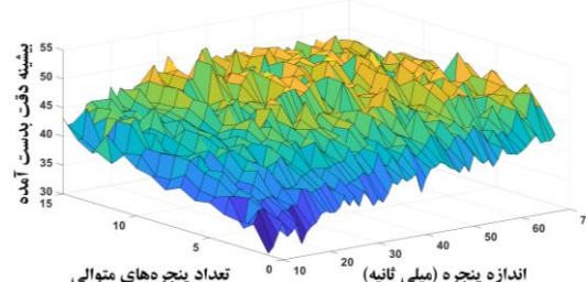
شکل ۷: بیشترین دقت بدست آمده در صورت تغییر متغیرهای طول محاسبه پنجره آتش و تعداد نرخ‌های آتش متوالی در فرآیند رمزگشایی روش پیشنهادی
