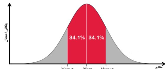
شکل ۴: سهم پراکندگی توزیع در یک توزیع نرمال
