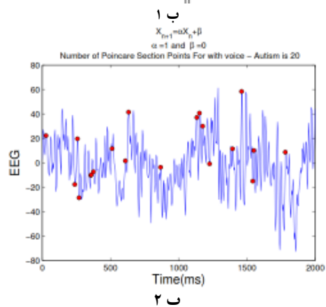
شکل ۱۰. قطع پوانکاره سیگنال EEG با خط Y=X در فضای بازسازی شده نسبی تگر و حوزه زمان الف. سالم ب. ASD
