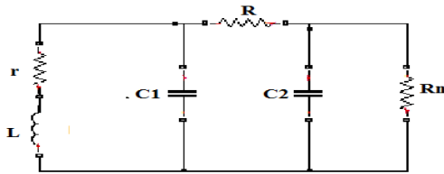
شکل ۱۰: مدل الکتریکی مدار چوا [۲۴].
