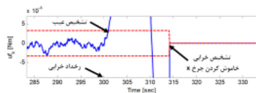
شکل ۱۴: تخمین اغتشاش چرخ عکس‌العملی (نمای نزدیک) در مود ۳
