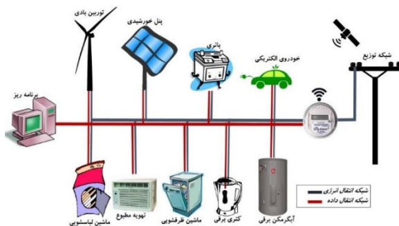
شکل ۳: اجزای نانوگرید مورد مطالعه
