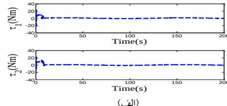
شکل ۱۴- خطاهای ردیابی e_3 و e_4 : (الف) کنترل کننده پیشنهادی (ب) کنترل کننده (۵۵)
