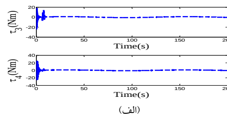
شکل ۱۵- ورودی های کنترل کننده اعمال شده به بدنه متحرک: (الف) کنترل کننده پیشنهادی (ب) کنترل کننده (۵۵)
