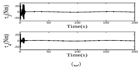
شکل ۱۶- ورودی های کنترل کننده مفاصل دو بازو: (الف) کنترل کننده پیشنهادی (ب) کنترل کننده (۵۵)
