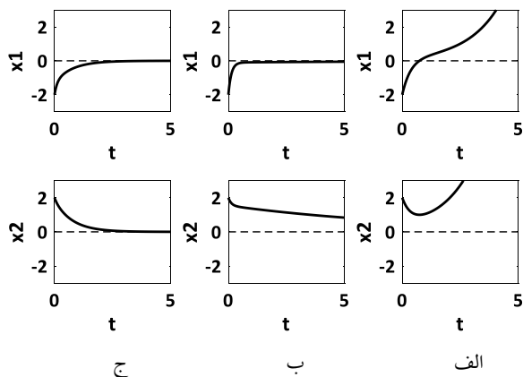
شکل ۳: مسیرهای حالت رسم شده به ازای شرط اولیه x_0 = [-2 \ 2]^T برای (الف) سیستم حلقه باز (ب) سیستم حلقه بسته پایدار شده توسط تابع لیاپانوف PWQ (پیوسته ج) سیستم حلقه بسته پایدار شده توسط تابع لیاپانوف PWQ ناپیوسته
