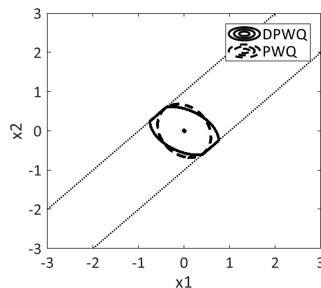
شکل ۵: ناحیه جذب سیستم حلقه باز به کمک تابع لیاپانوف PWQ ناپیوسته (خط ضخیم) و به کمک تابع لیاپانوف PWQ پیوسته (خط چین) با حل مسأله ۲، به ازای هر i \in I ، ضرایب کنترل کننده فیدبک حالت \bar{M}_i و ماتریس‌های \bar{P}_i متناظر با تابع لیاپانوف PWQ پیوسته به صورت زیر بدست آمده است:
