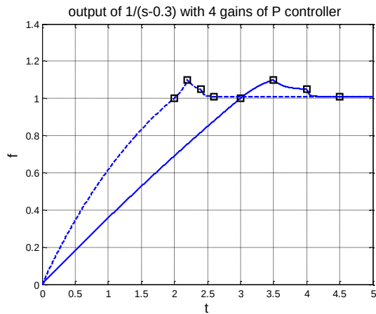
شکل ۱۹- نمودار خروجی سیستم \frac{1}{s-0.3} با چهار بهره‌ی متغیر با زمان کنترل کننده‌ی تناسبی
