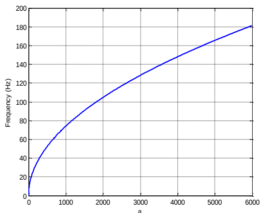
شکل ۸: نمودار منحنی فرکانس به ازای مکان قطب کنترل کننده (حالت اول)
