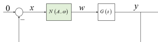
شکل ۲: سیستم خطی همراه با تابع توصیفی عنصر غیرخطی
