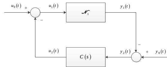
شکل (۲): بلوک دیاگرام استاندارد سیستم کنترل غیرخطی حلقه بسته با کنترل کننده خطی
