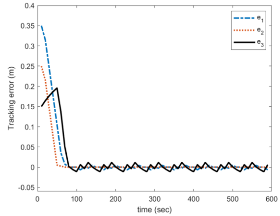
شکل ۷: خطای ردیابی
