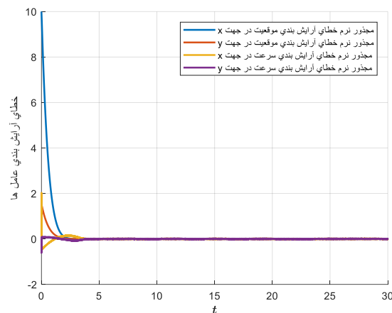
شکل ۱۲- نمایش خطای آرایش‌بندی عامل‌ها در حضور اغتشاش
