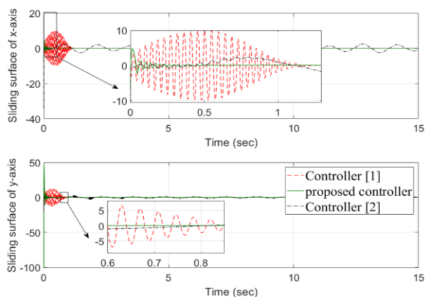
شکل ۹: تحول زمانی عملکرد روتینگر در تخمین سرعت‌ها
