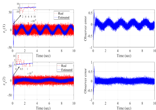
شکل ۱۰: نتایج عملکرد روتینگر هوشمند در تخمین مجموع نامعینی‌ها
