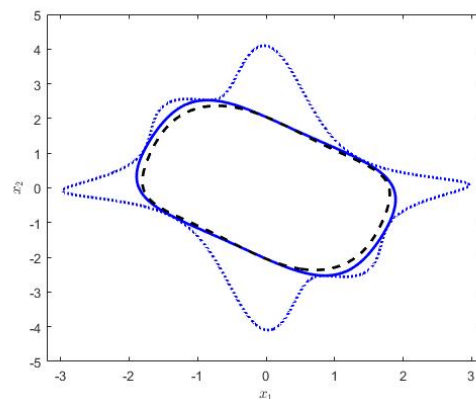
شکل ۶: منحنی سیاه خط چین تخمین ناحیه جذب بر اساس فیدبک حالت [۲۲]، منحنی آبی خط پیوسته تخمین DA با روش پیشنهادی، منحنی آبی نقطه چین \dot{V}(x) = 0
