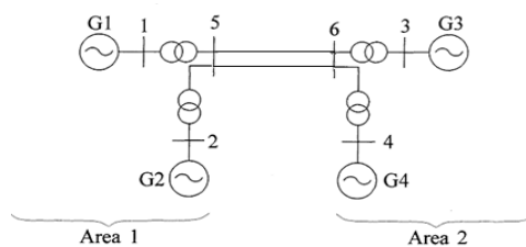
شکل ۱: سیستم ۴ ژنراتور و خط ۵
