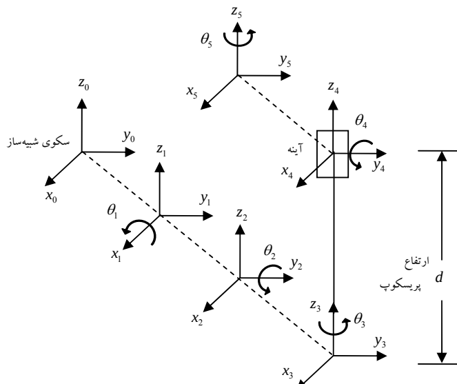
شکل ۳: سیستم مختصات پریسکوپ متصل به سکوی شیشه ساز
