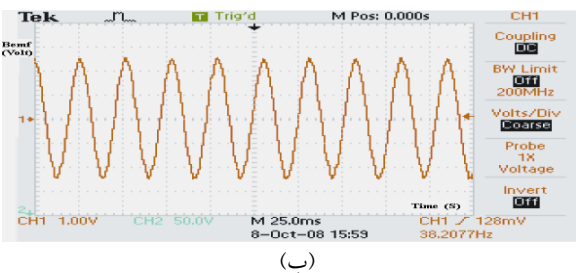
شکل ۴. الف. ولتاژ Back-EMF القا شده در سیم‌پیچی استاتور. الف. شبیه‌سازی شده با مدل MEC. ب. نتیجه‌ی عملی با نسبت ۱ به ۱۰.
