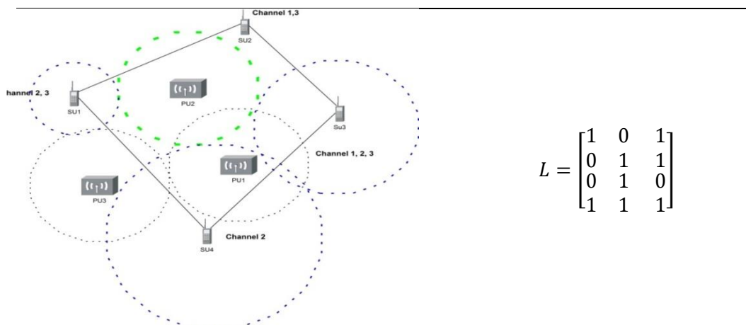
شکل ۱. یک شبکه رادیوی شناختگر با ۳ کاربر اولیه و ۴ کاربر ثانویه ناحیه تحت پوشش این کاربران و ماتریس دسترسی‌پذیری آن
