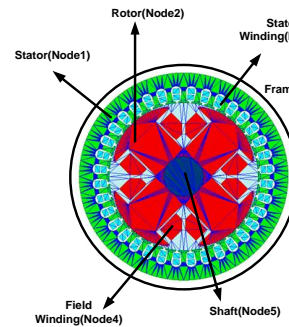
شکل ۴: گره بندی ژنراتور سنکرون به منظور محاسبه خازنهای پارازیتی
