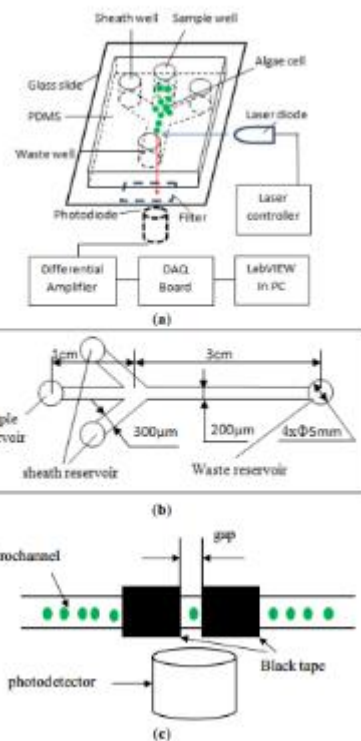
شکل ۴: ساختار کلی تشخیص سلول زنده و مرده
