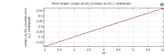
شکل ۳۸: نمودار مربوط به تغییرات میزان خازن شانه ای بر حسب تغییرات تعداد شانه ها
