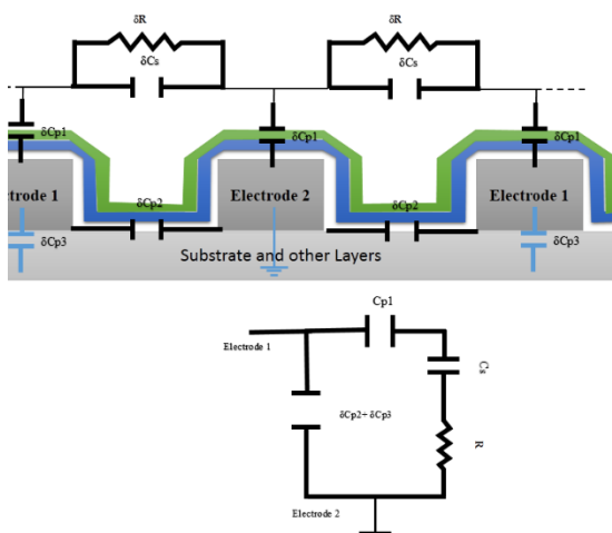
شکل ۶۲: (a) خازن های پارازیتی ایجاد شده بر روی تراشه ی CMOS و \delta C و \delta R به ترتیب خازن با پارازیت جزئی ۳ و مقاومت هستند. و (b) مدار معادل ۴ کل میکرو ساختار است.
