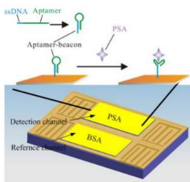
شکل ۷: میکرو ساختار حسگر تشخیص آنتی ژن پروستات در [۳۵] یک حسگر آپتامری و ریزسیالی بر مبنای تغییر امپدانس خروجی جهت تشخیص ویروس آنفولانزا معرفی شده است.
