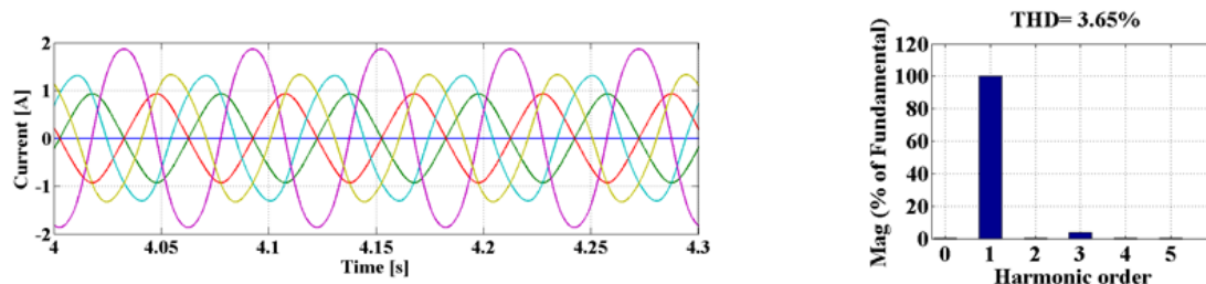
شکل ۷: شکل موج جریانهای موتور در حالت قطع فاز \alpha_1 و هارمونیک جریان فاز \beta_1 با کنترل کننده ADRC
