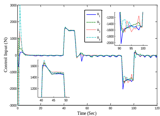
شکل ۱۱: ورودی کنترلی در سناریو ۱، استراتژی فاصله ثابت
