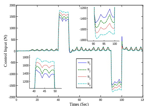
شکل ۱۶: ورودی کنترلی برای سناریو ۲، استراتژی زمان پیشرفت ثابت
