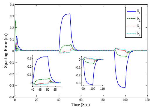
شکل ۱۳: خطای تعقیب برای سناریو ۱، استراتژی زمان پیشرفت ثابت
