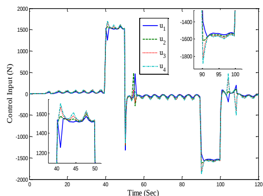
شکل ۱۵: ورودی کنترلی در سناریو ۱، استراتژی زمان پیشرفت ثابت
