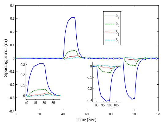
شکل ۱۴: خطای تعقیب در سناریو ۲، استراتژی زمان پیشرفت ثابت
