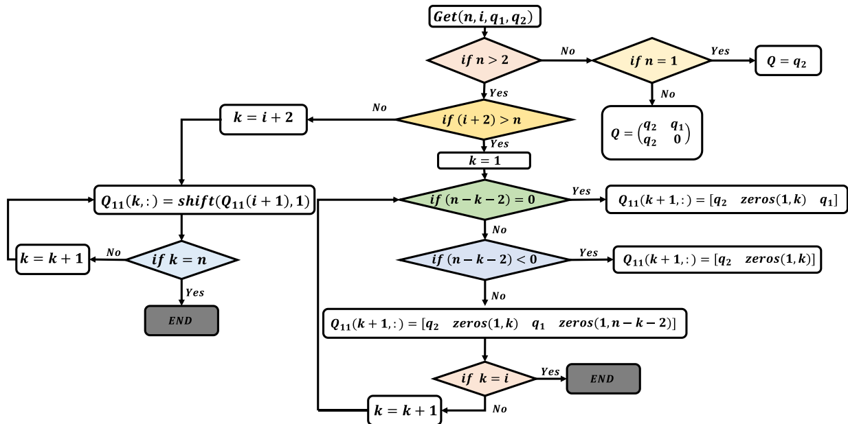
شکل ۵: فلوچارت پیشنهادی برای استخراج ماتریس Q_{11}
