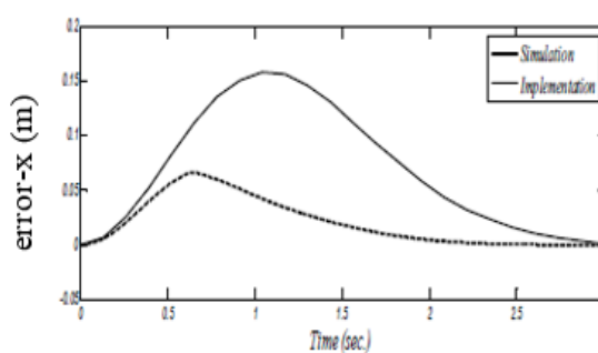
(پ) خطای حرکتی در راستای محور X
