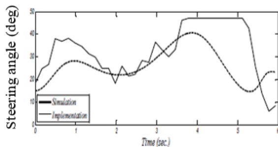
(ج) زاویه هدایت فرمان ربات شبه‌خودرو
