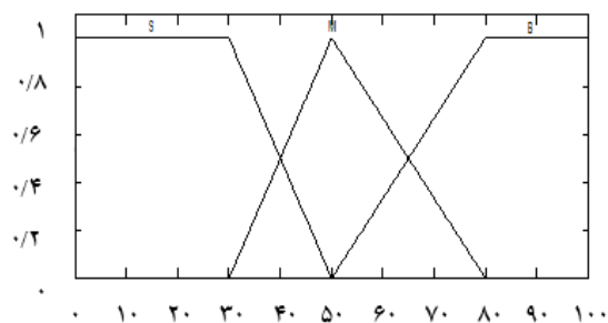
(ت) توابع عضویت سرعت خودروهای در حال حرکت (m/s)
