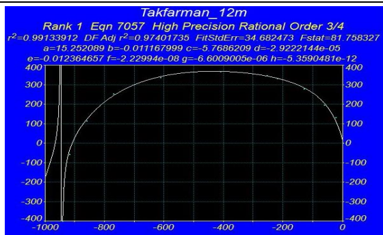
شکل ۲: برازش اطلاعات مسیر خیابان ۱۲ متر
