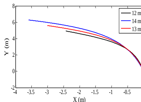
شکل ۴: درون‌یابی مسیر رفت دوزدن تک‌فرمان خیابان ۱۳ متر
