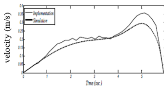
(ث) سرعت ربات شبه‌خودرو
