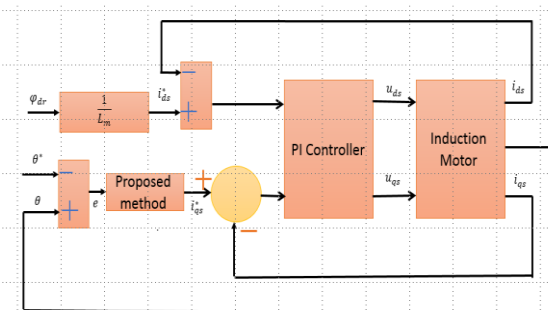
شکل ۱- بلوک دیاگرام سیستم کنترل
