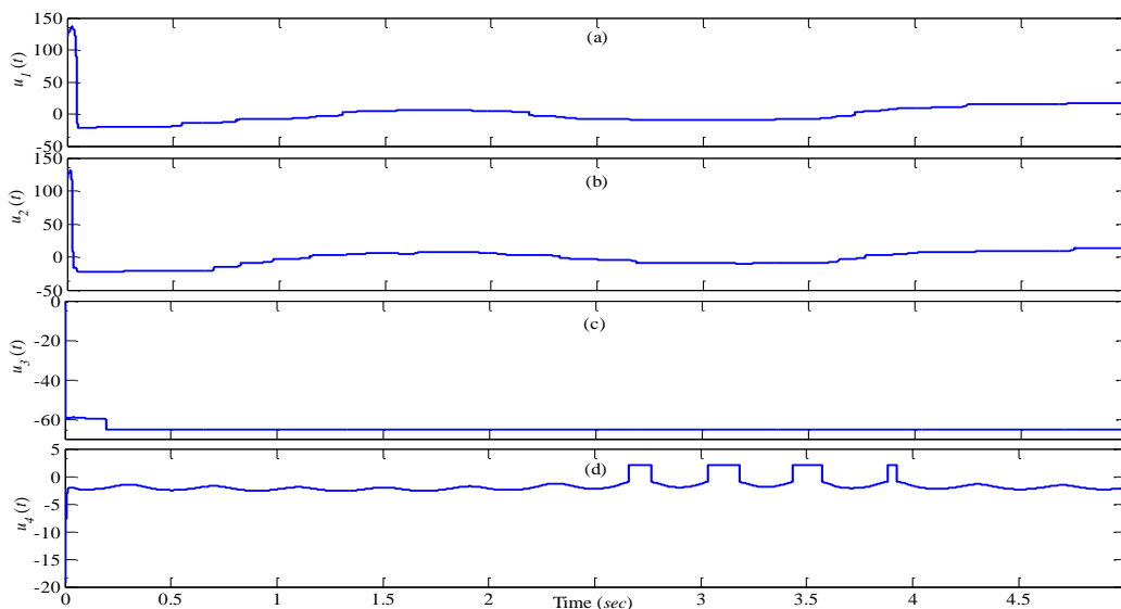
شکل ۱۱. پاسخ‌های زمانی گشتاورهای پیشنهادی دسته چهارم با فرض در نظر گرفتن غیرخطی‌سازهای ناحیه مرده. (a): پاسخ زمانی u_1(t) ; (b): پاسخ زمانی u_2(t) ; (c): پاسخ زمانی u_3(t) و u_4(t) ; (d): پاسخ زمانی u_4(t)
