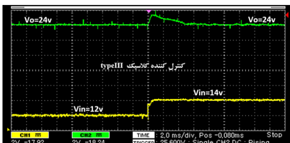
شکل (۱۵) - پاسخ عملی میدل پست در شرایط تغییر ولتاژ ورودی مربوط به کنترل کننده کلاسیک typeIII و کنترل کننده بهینه مبتنی بر جواب شماره ۸ از جبهه پاراتو typeIII+PIDWCZ
