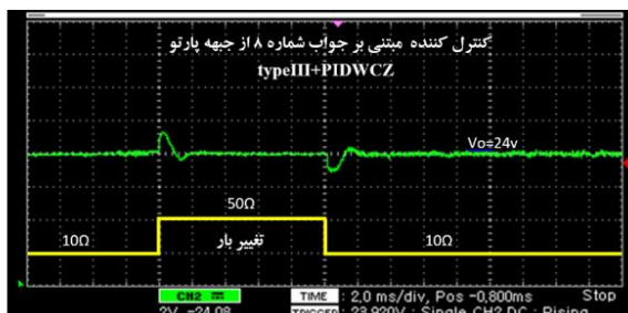
شکل (۱۳) - پاسخ عملی میدل پست در شرایط تغییر بار مربوط به کنترل کننده کلاسیک typeIII و کنترل کننده بهینه مبتنی بر جواب شماره ۸ از جبهه پاراتو typeIII+PIDWCZ
