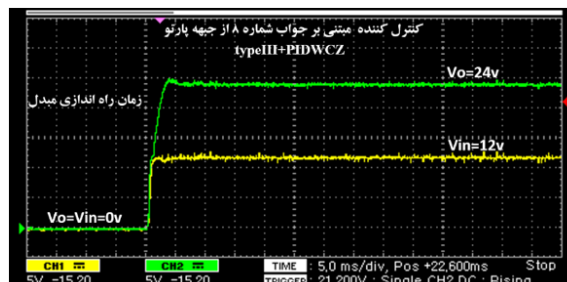
شکل (۱۲) - پاسخ عملی میدل پست در شرایط راه اندازی مربوط به کنترل کننده کلاسیک typeIII و کنترل کننده بهینه مبتنی بر جواب شماره ۸ از جبهه پاراتو typeIII+PIDWCZ
