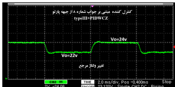
شکل (۱۴) - پاسخ عملی میدل پست در شرایط تغییر ولتاژ مرجع مربوط به کنترل کننده کلاسیک typeIII و کنترل کننده بهینه مبتنی بر جواب شماره ۸ از جبهه پاراتو typeIII+PIDWCZ
