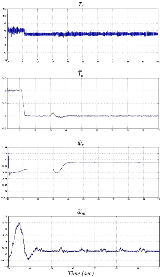
شکل ۶: عملکرد موتور فقط با وجود کنترل کننده نامی در حضور خطای مکانیکی استاتور
