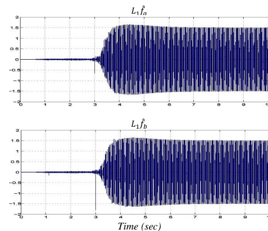
شکل ۷: تخمین خطاهای جمع شونده ناشی از خطای مکانیکی استاتور توسط رویکرد
