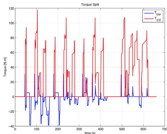
شکل ۱۴: تقسیم گشتاور بین موتورهای الکتریکی و درونسوز
