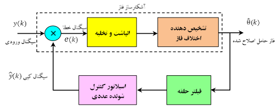
شکل ۳: مورو بر معماری PLL سنتی همراه با بلوکهای سازنده آن [۷]
