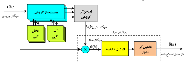
شکل ۷: روش حلقه باز برای ردیابی سگنال حامل [۳۸،۳۹].
