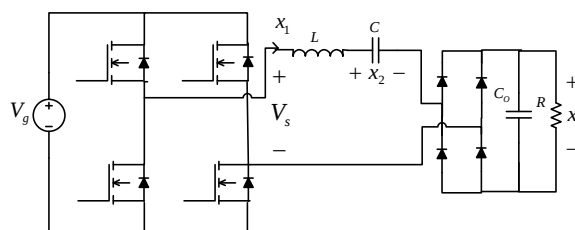
شکل ۴: مبدل الکترونیک قدرت dc-dc رزونانسی سری
