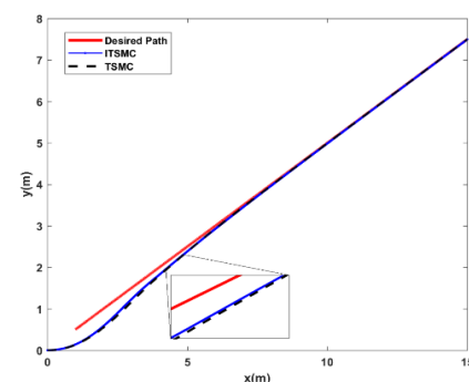
شکل ۱۲: مسیر مستقیم طی شده و مسیر مطلوب شناور در دو بعد
