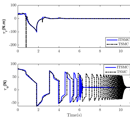
شکل ۱۱: خروجی‌های کنترلی شناور
