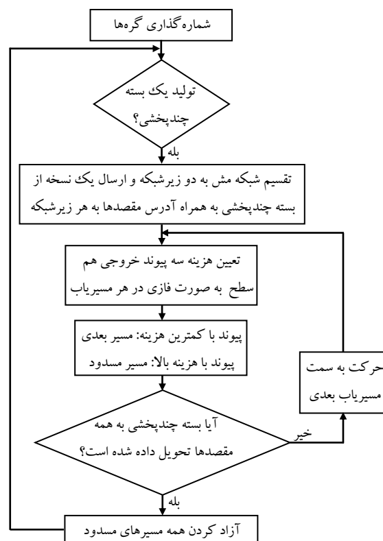
شکل ۴: فلوچارت الگوریتم مسیریابی پیشنهادی (MARFA)
