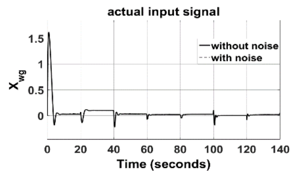
شکل ۲۳: باز شدن واقعی در پیچه برای مدل غیرخطی با و بدون نویز
