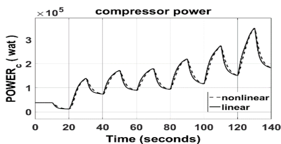
شکل ۹: توان کمپرسور برای مدل غیر خطی و خطی
