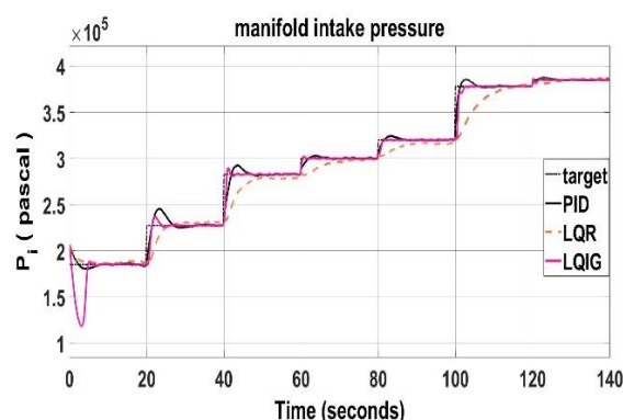
شکل ۱۳: مقایسه خروجی کنترل‌کننده‌های PID، LQR و LQIG
