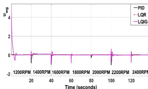
شکل ۱۴: مقایسه سیگنال کنترل کنترلگرهای PID، LQR و LQIG
