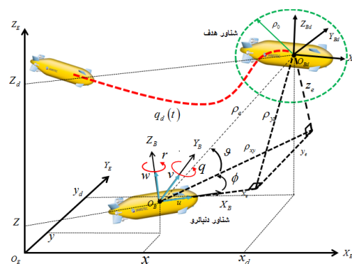
شکل ۱: ردیابی هدف زیردریایی در فضای سه بعدی [۲۹]
