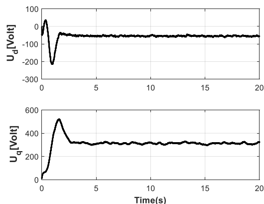
شکل ۳- سیگنال‌های کنترلی اعمال شده به سیستم نامی
