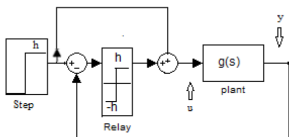
شکل ۵. بلوک دیاگرام تست رله اصلاح شده
