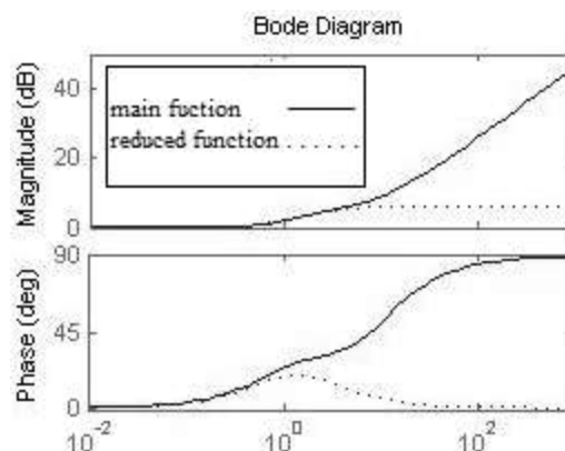
شکل ۲. نمودار بود برای تابع تبدیل ناسره و تابع تبدیل سره شده با حذف صفر بزرگ
