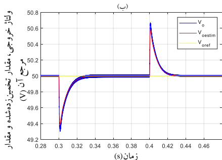
شکل ۴. رگولاسیون: (الف) جریان سلف، مقدار تخمین زده شده و مرجع آن (ب) شکل موج ولتاژ خروجی، مقدار تخمین زده شده و مرجع آن، با تغییر مقدار مقاومت با از ۴۸ اهم به ۲۴ اهم در زمان ۰/۳ ثانیه و از ۲۴ اهم به ۴۸ اهم در زمان ۰/۴ ثانیه.
