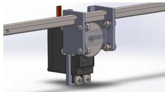
شکل ۳ طرح مفهومی از دوبره کنترل شونده از طریق جابجایی مرکز جرم
